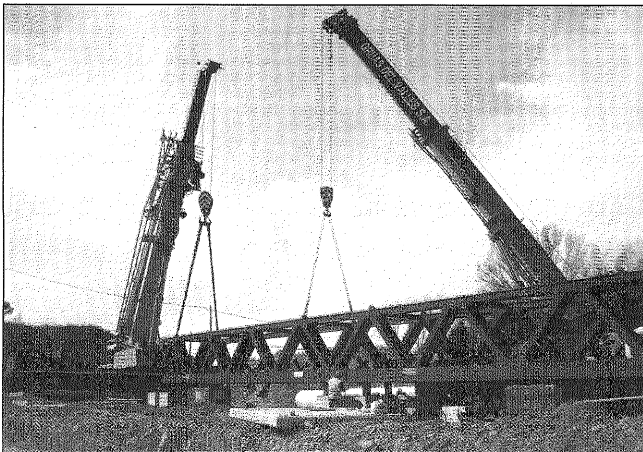
El cos central de l'estructura ha arribat a Sant Celoni aquest dilluns i s'ha procedit a instal·lar-la (AdBM)
