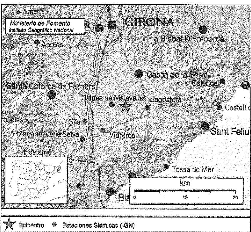
Mapa de l'episodi sísmic elaborat per l'Institut Geográfico de l'Estat (AdBM)
